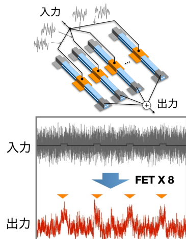
生物機能である確率共鳴を電子デバイス上で再現
